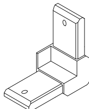
Aplicação no contramarca, nos perfis CM200 e CM151
