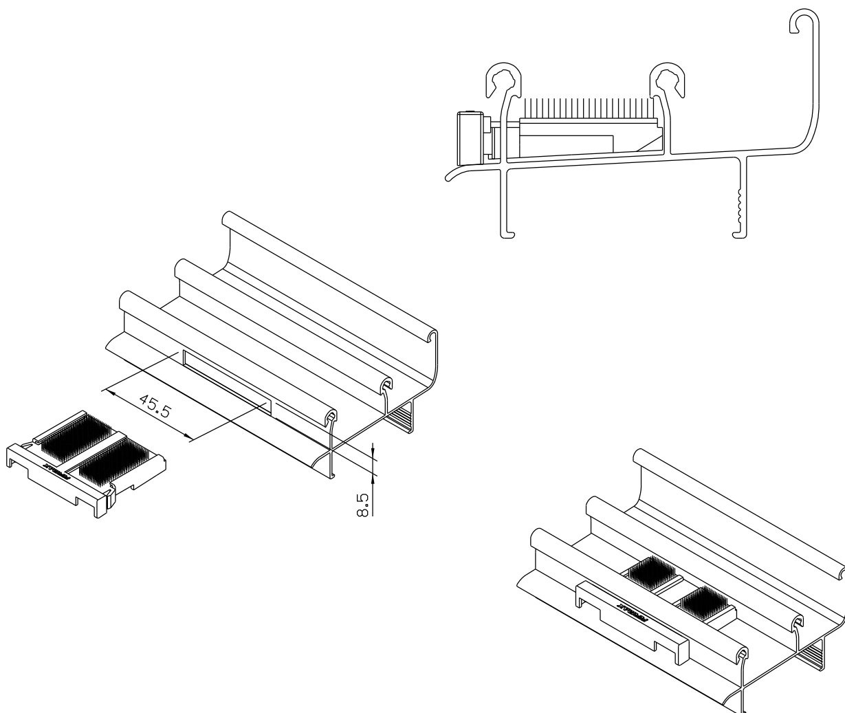
DETALHE DE APLICAÇÃO - sem escala
