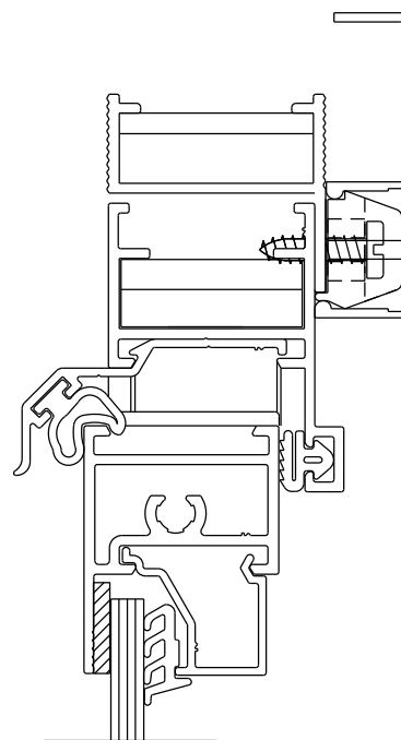
Instalação - escala 1:1
