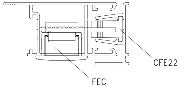
contra-fecho lateral
