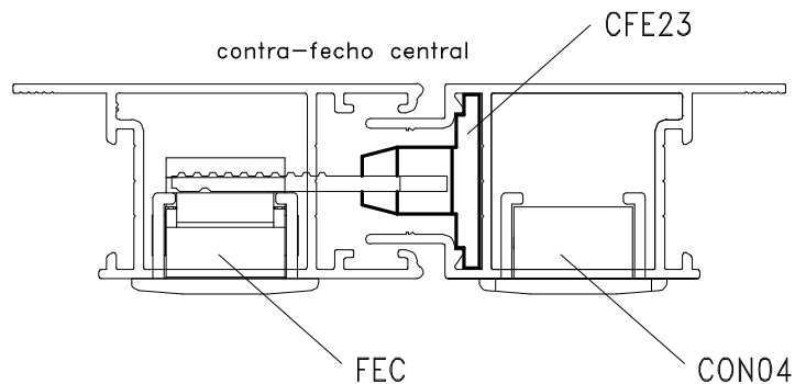
Instalação - escala 1:1
