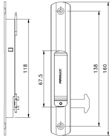
Vistas - escala 1:2
