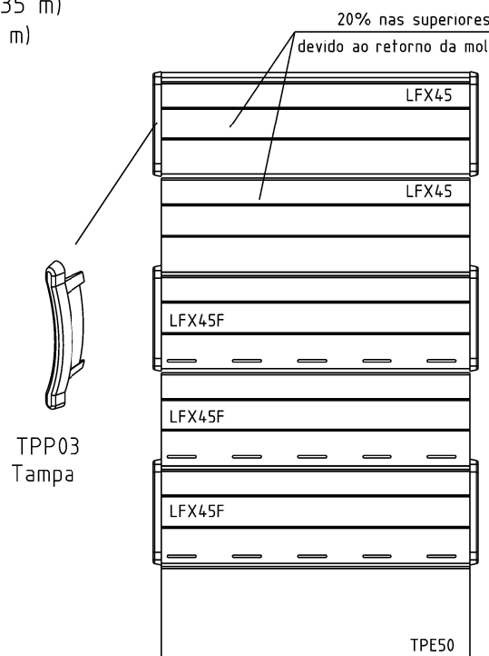
Orientação de montagem
