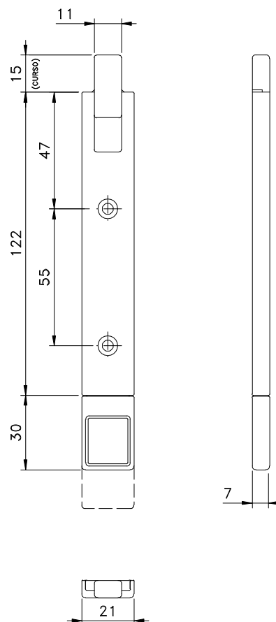
Vistas — escala 1:2
