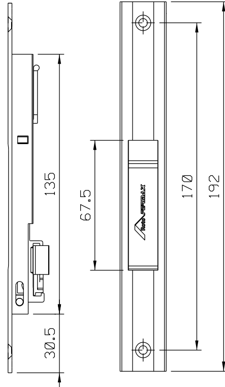
Vistas - escala 1:2
