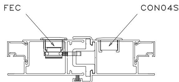
Instalação - escala 1:1
