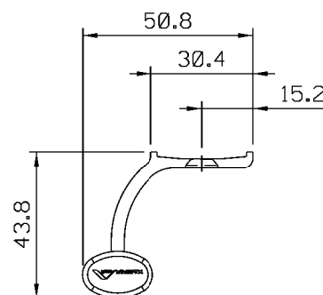
Vistas - escala 1:2
