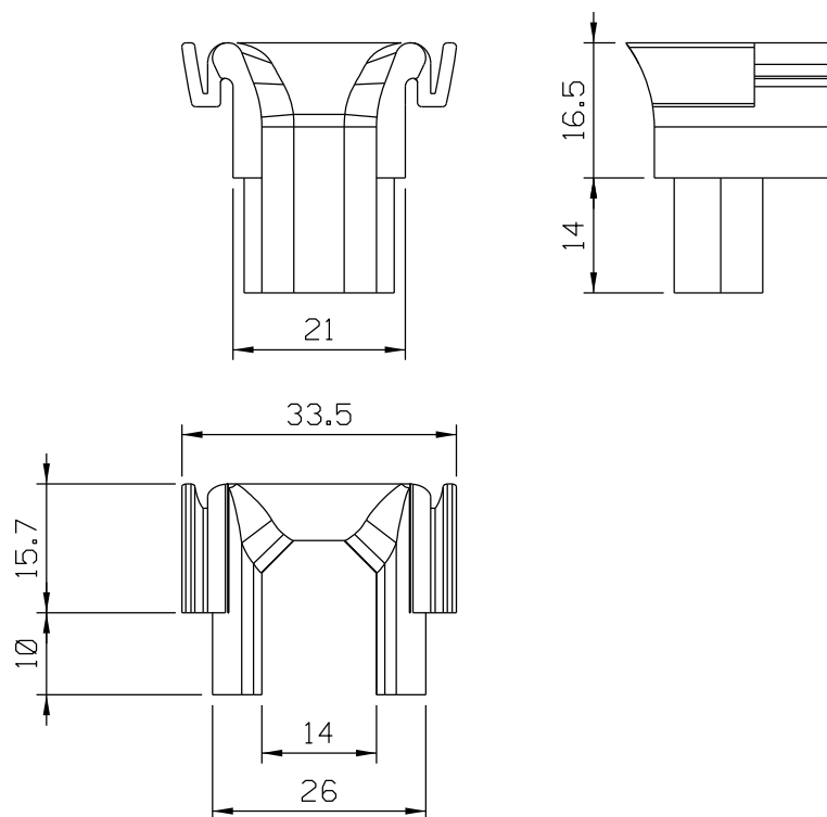
Vistas - escala 1:1
