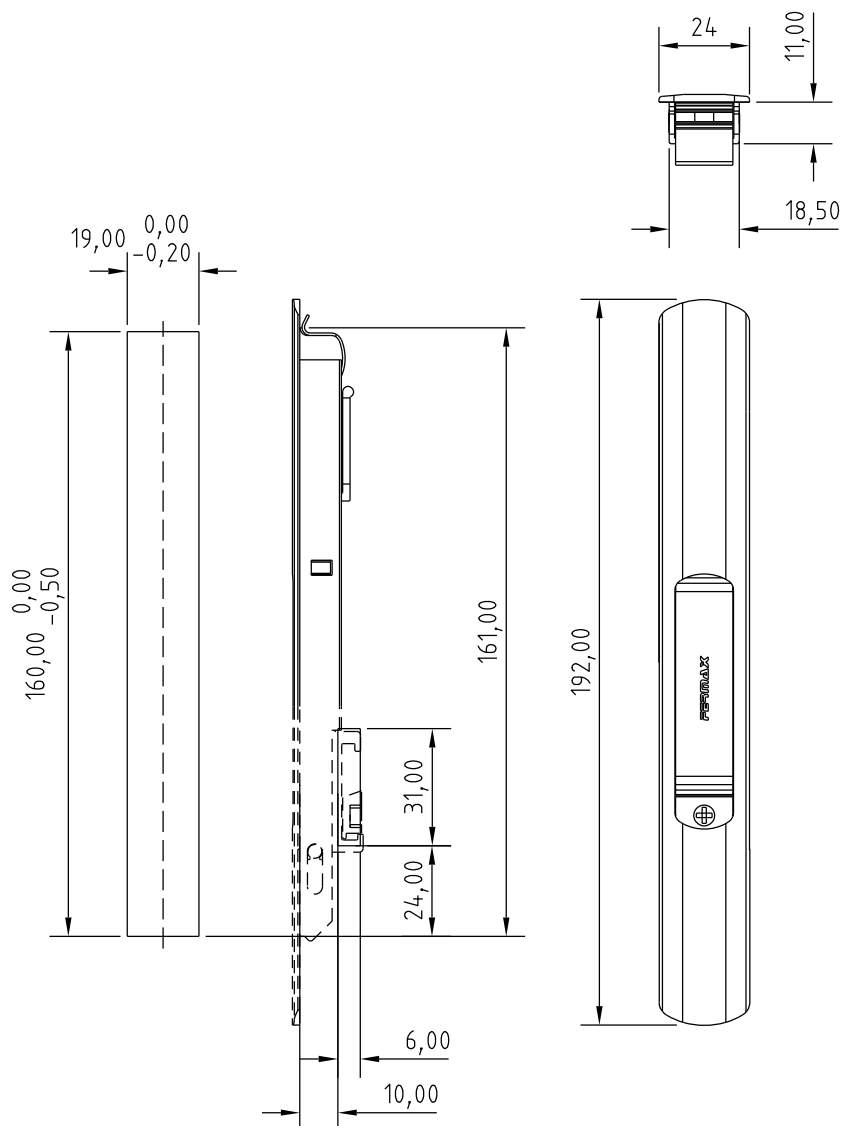
USINAGEM – escala 1:2
