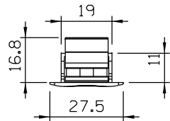
Vista - escala 1:2
