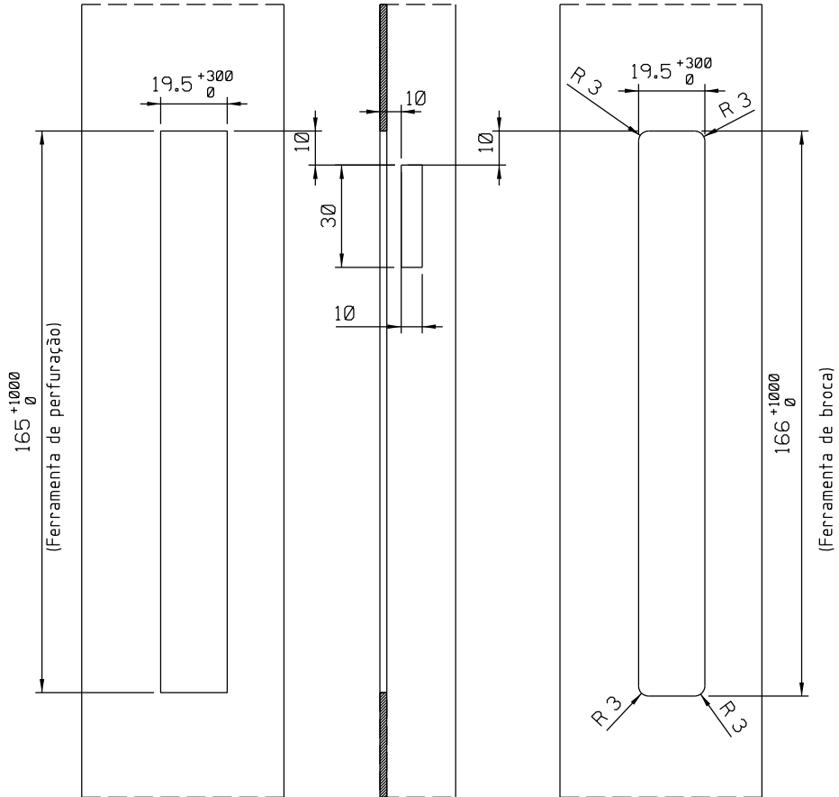
Usinagem - escala 1:2
