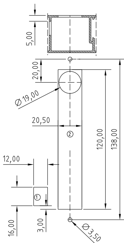
USINAGEM - ESCALA 1:2
