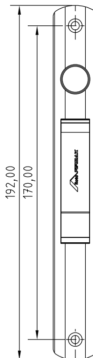
VISTAS - ESCALA 1:2
