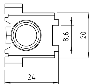
VISTAS ESCALA 1:1
