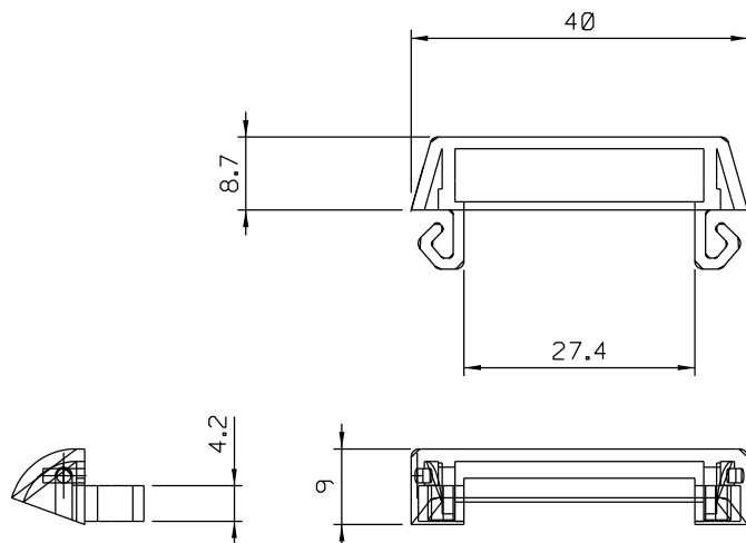
VISTAS ESCALA 1:1
