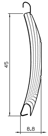
Vista - escala 1:1
