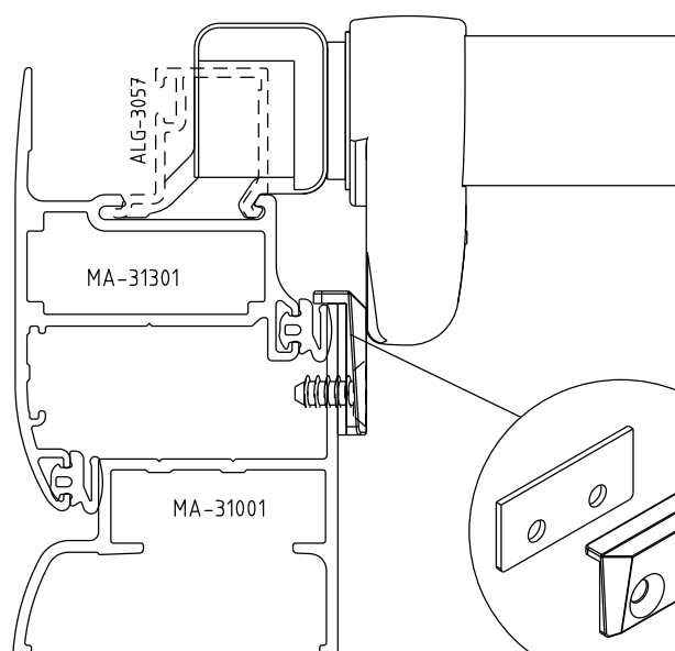
INSTALAÇÃO - ESCALA 1:1
