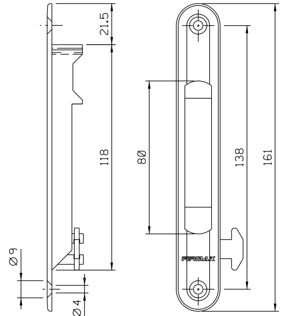
Vistas - escala 1:2
