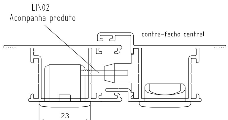
Instalação - escala 1:1
