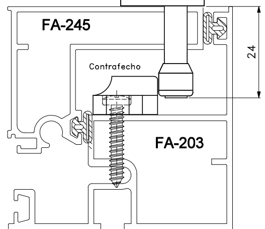
Instalações - escala 1:1
