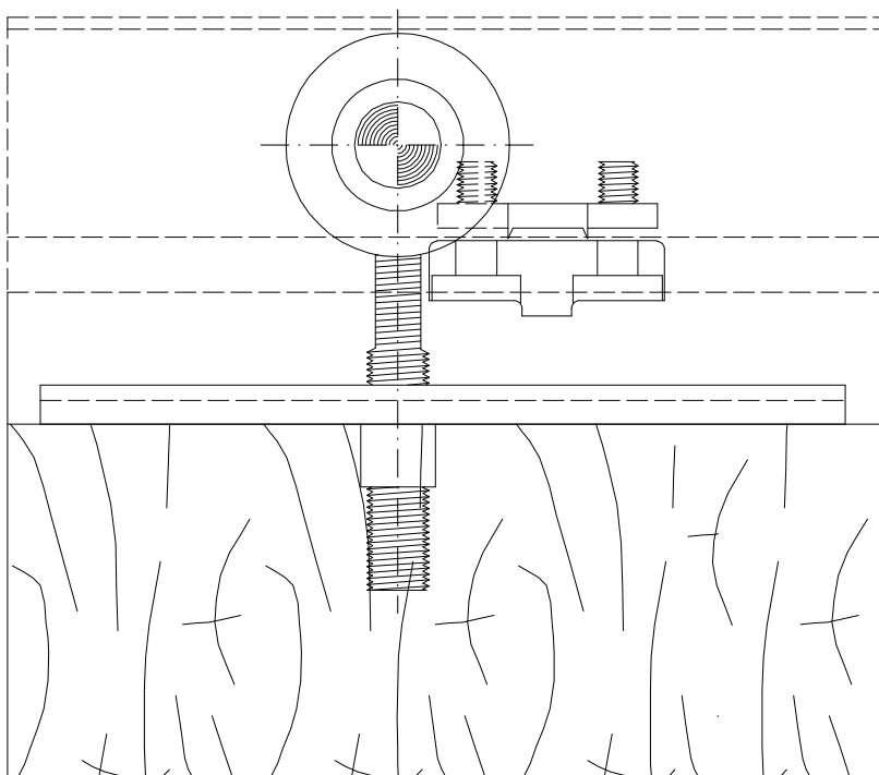
DETALHE DE INSTALAÇÃO Escala: 1:1
