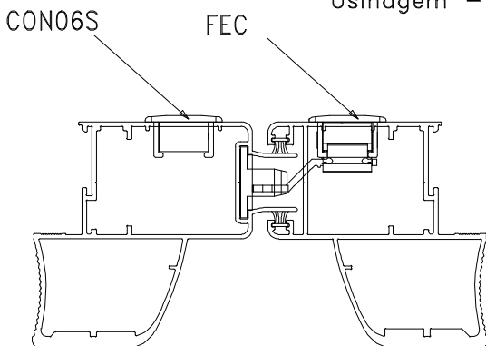
Usinagem - escala 1:1
