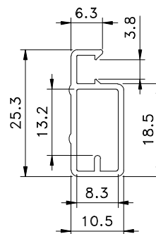
Vista — escala 1:1
