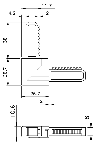
Vistas — escala 1:2
